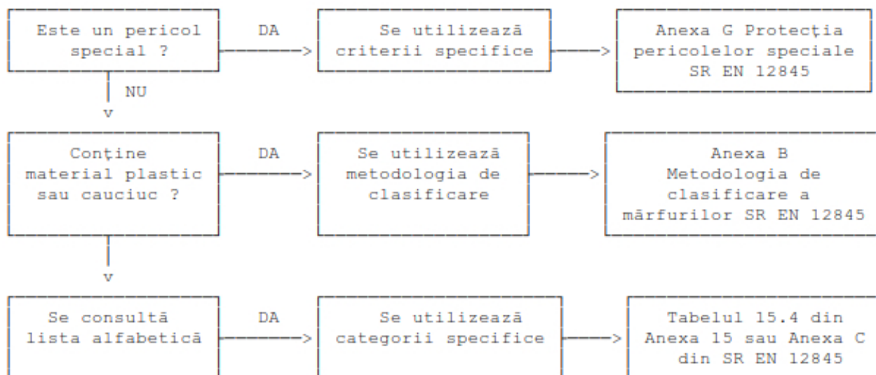
Figura 7.2. Schemă de determinare a claselor de pericol la incendiu pentru depozite (conform SR EN 12845)
