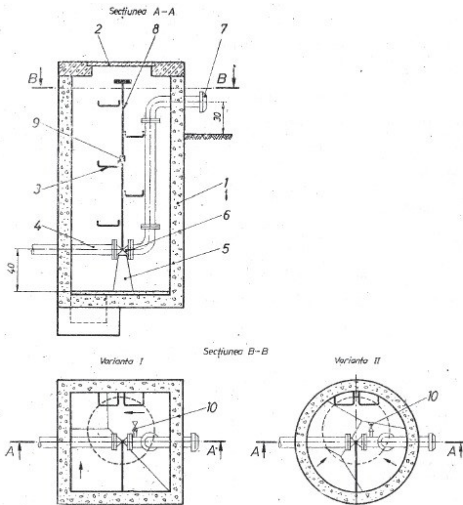
Figura. 12.2 Cămin de alimentare directă cu apă a pompelor mobile de tip B
