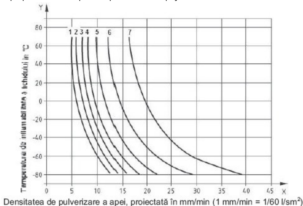
Figura. 8.1 Densitatea de pulverizare a apei pentru stingerea incendiilor de produse petroliere vărsate, pe baza punctelor de inflamabilitate a lichidului. Curbele 1, 2, 3, 4, 5, 6 și 7 corespund pentru înălțimi ale tavanului mai mici respectiv de 3m, 4m, 5 m, 6m, 7m, 8 m și 9m.
