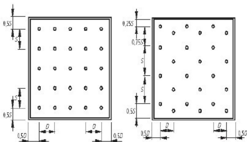
Figura 7.5. Distanțele maxime S și D de amplasare (dispunere) a sprinklerelor, în plan orizontal, sub tavan: a - amplasare (dispunere) standard (în rânduri paralele); b - amplasare (dispunere) în zig-zag
