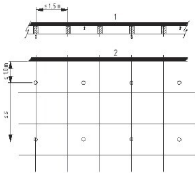
Figura 7.7 Amplasarea sprinklerelor pe traveele drepte formate între grinzile așezate pe două direcții, la distanța sub 1,5 m: 1 - tavan; 2 - perete
