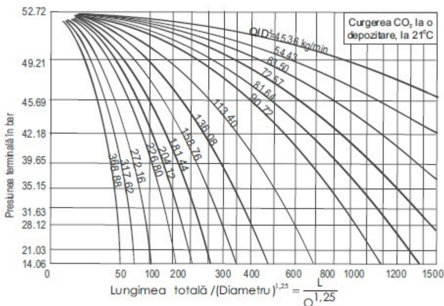
Figura 16.3. - Nomogramă pentru calculul de verificare a debitelor de curgere a dioxidului de carbon în conductele instalațiilor de joasă presiune (presiunea de depozitare a CO(2) de 20,7 bar la temperatura de 21°C).
