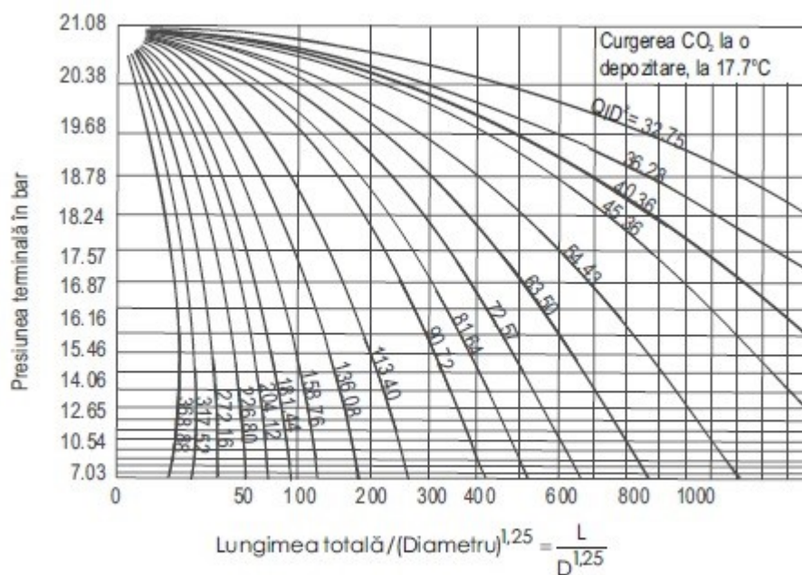
Figura 16.2. - Nomogramă pentru calculul de verificare a debitelor de curgere a dioxidului de carbon în conductele instalațiilor de înaltă presiune (presiunea de depozitare a CO(2) de 51,7 bar la temperatura de 17,7°C).
