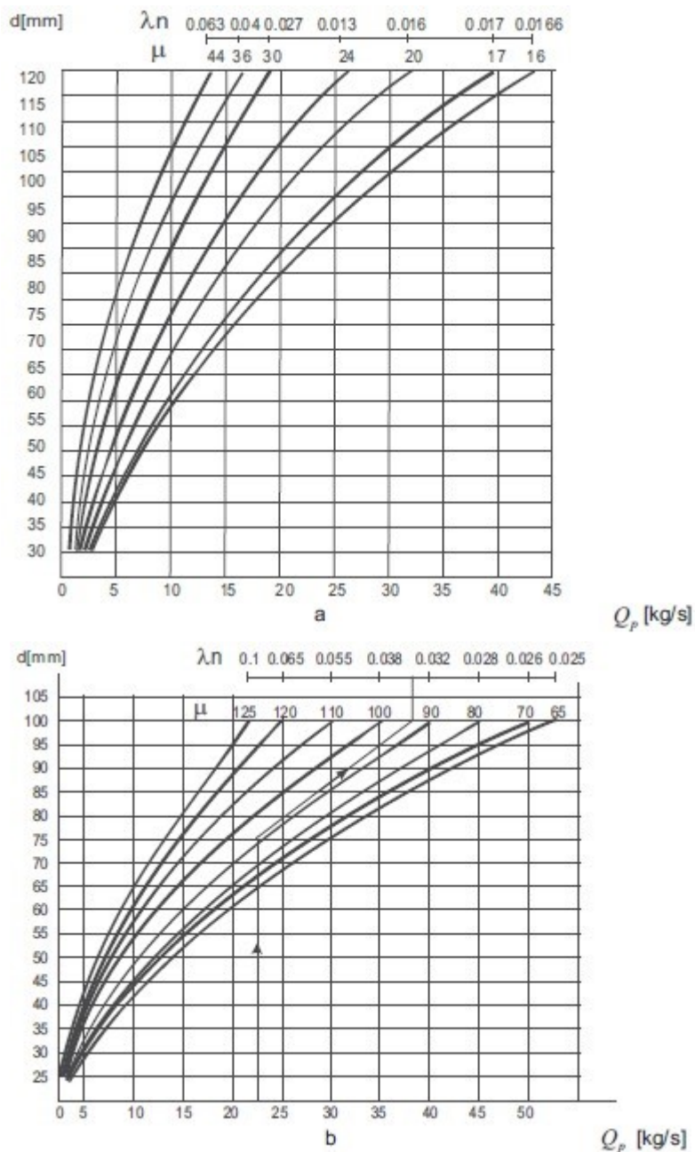
Figura 26.1. Nomograme de dimensionare a conductelor principale de transport a pulberii: a - pentru \lambda(n) = 0,0166 \dots 0,063 ; b - pentru \lambda(n) = 0,025 \dots 1
