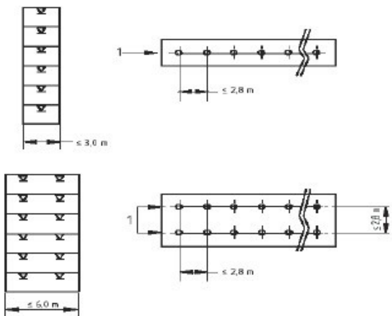
Figura 7.11 Amplasarea sprinklerelor intermediare pentru tipurile de depozitare ST5 și ST6: 1 - rând de sprinklere
