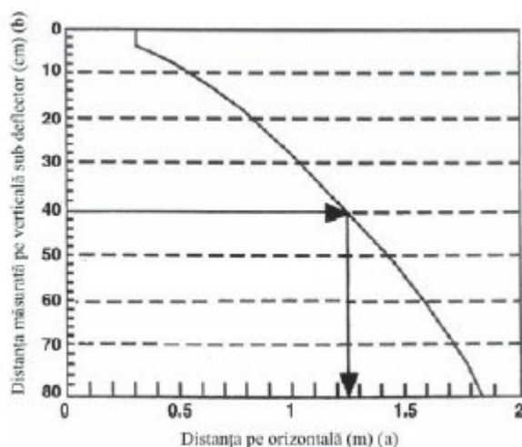
Figura 7.17 - Nomogramă de stabilire a distanțelor de amplasare a sprinklerelor față de elementele vecine
