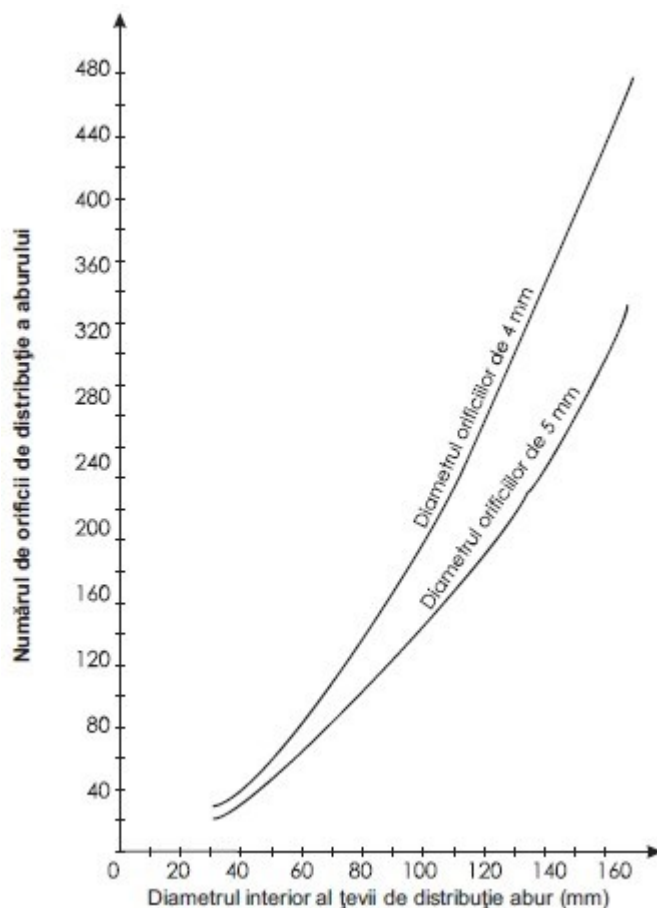
Figura 27.1. Nomogramă pentru determinarea numărului de orificii de ieșire a aburului pentru stingerea incendiului.
