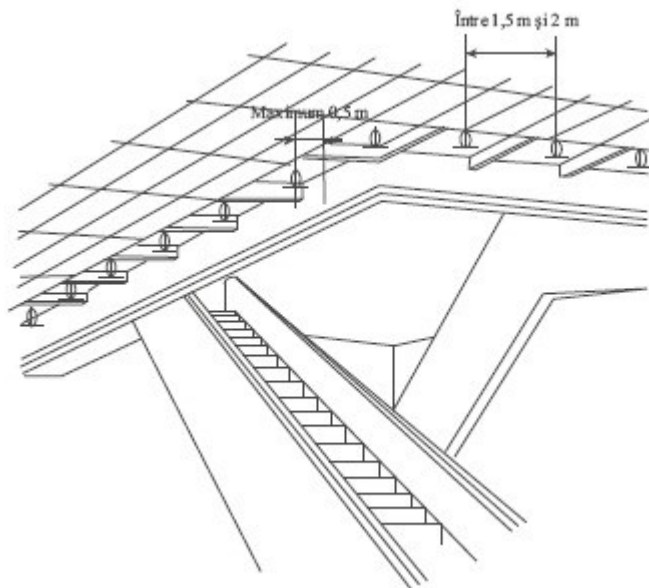
Figura 7.10 Amplasarea sprinklerelor în jurul golurilor din tavane
